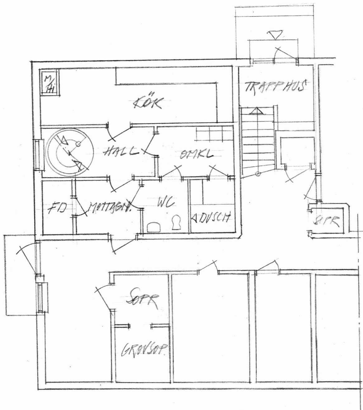
KÄLLARPLAN 1:100
